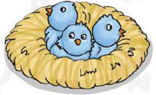
NEST
